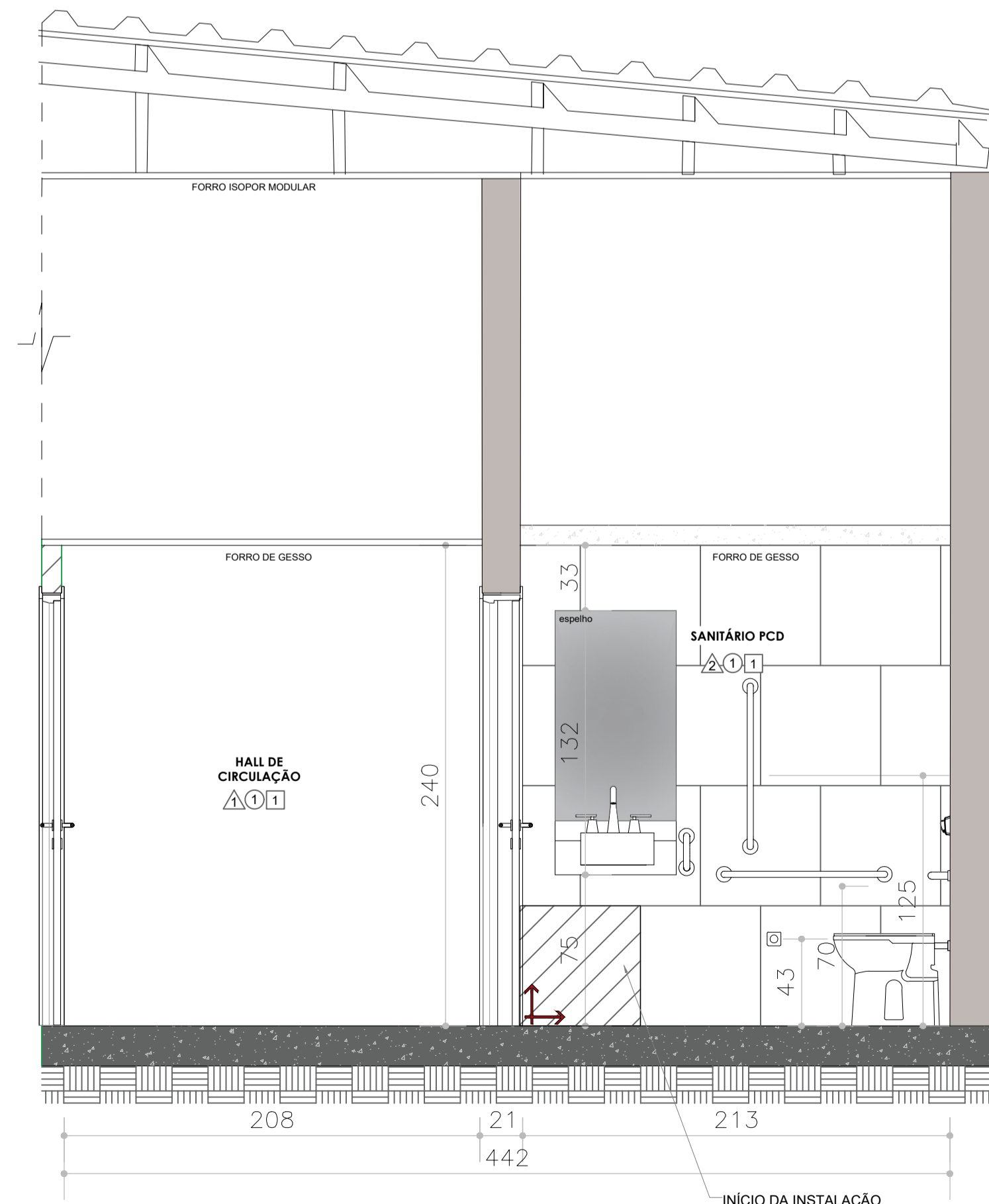
14 CORTE F-F ESCALA 1:25
