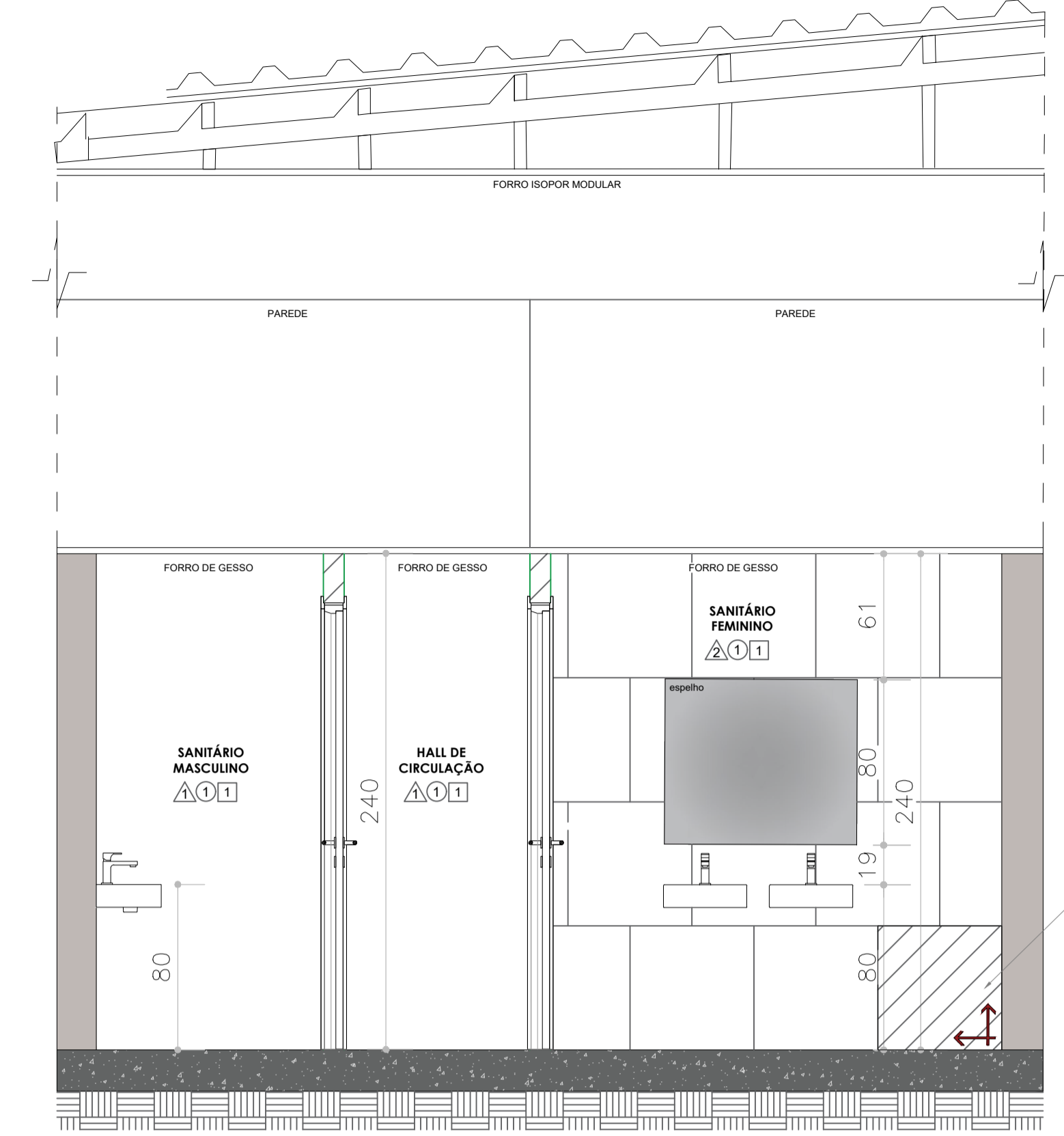
13 CORTE E-E ESCALA 1:25
