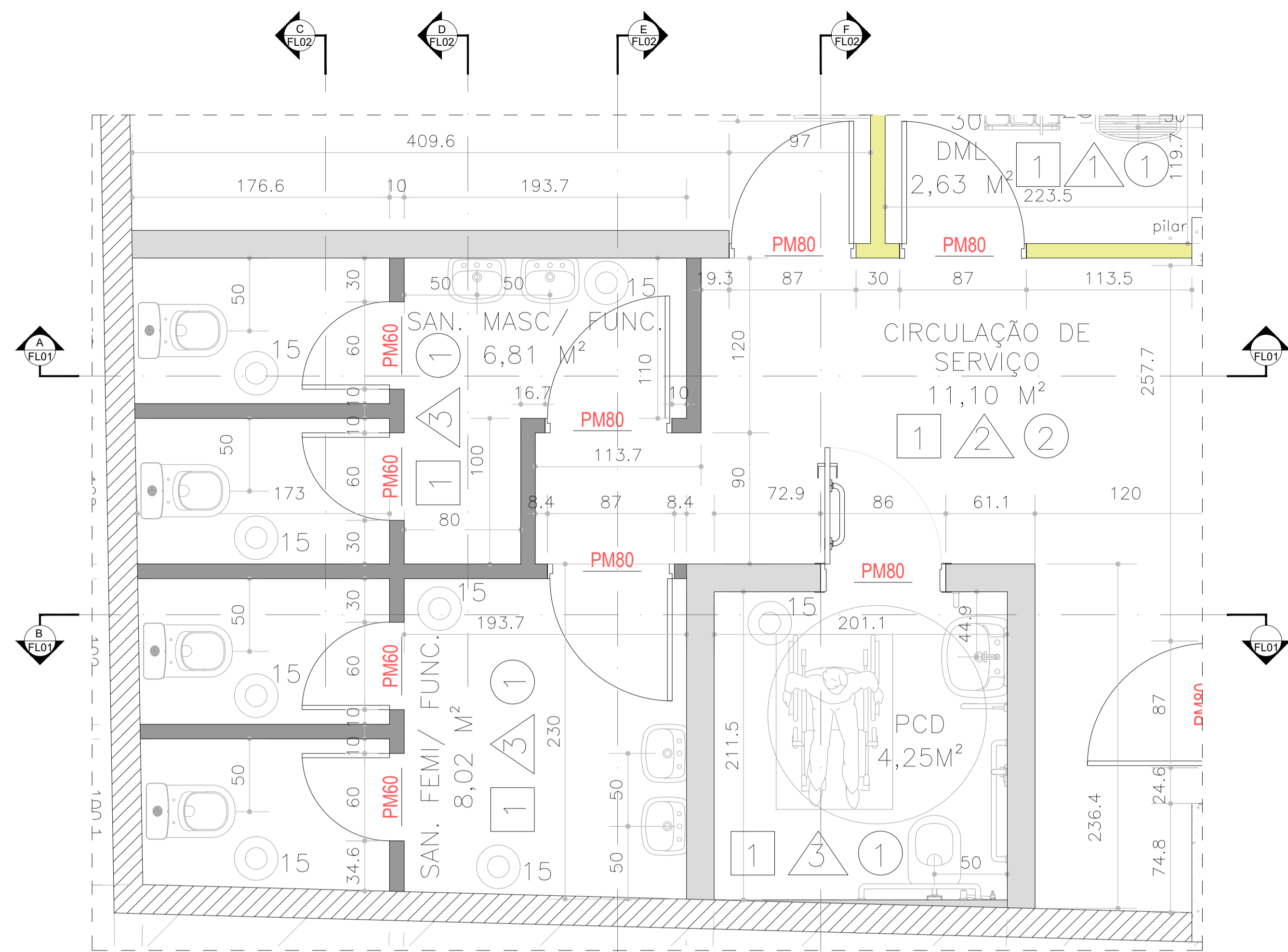
08 PLANTA BAIXA - SANITÁRIOS ESCALA 1:25
