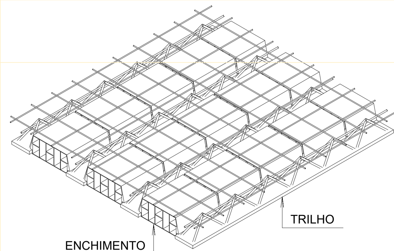
DETALHES DA LAJE SEM ESC.
