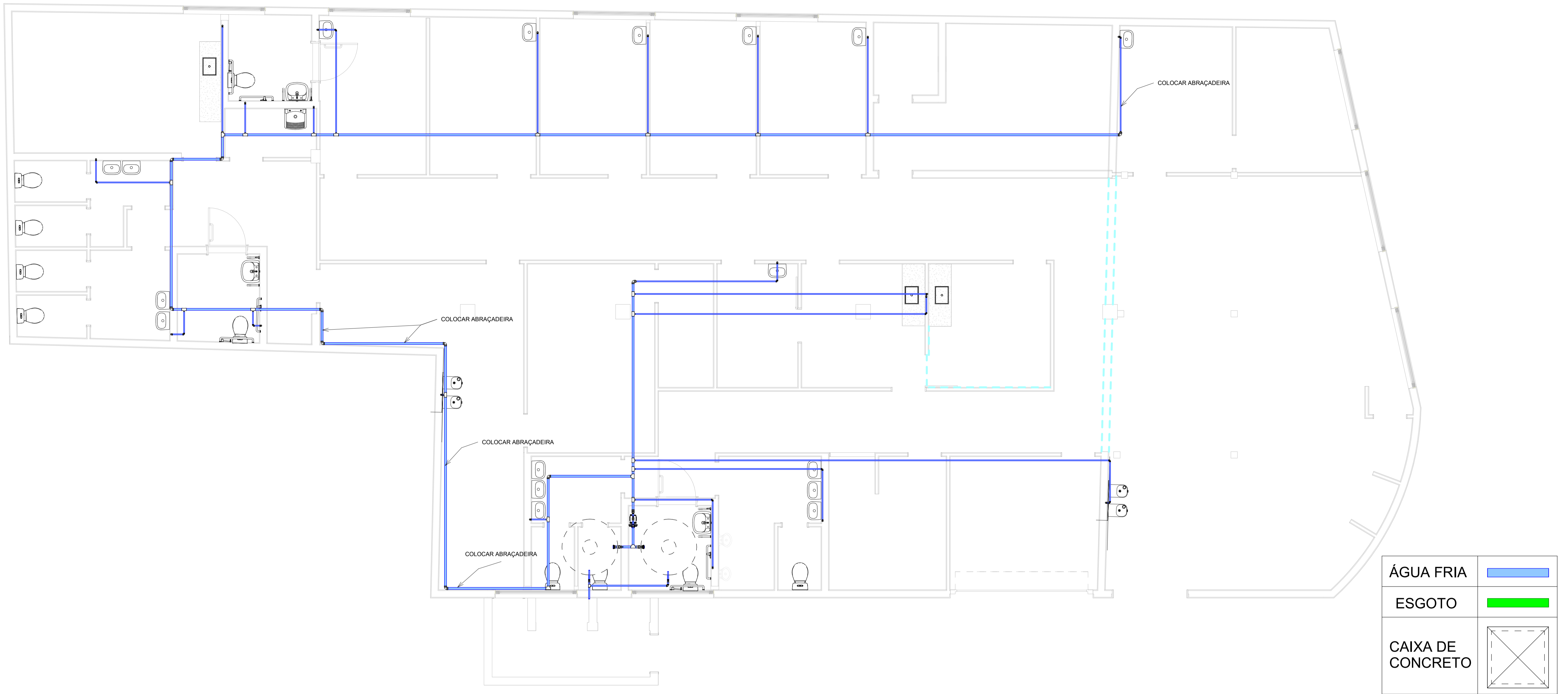
17 PLANTA BAIXA 1 : 50
