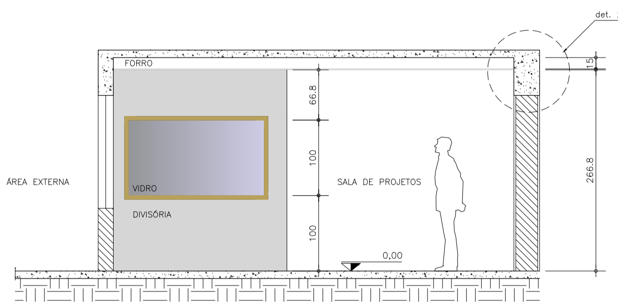
CORTE A VISTA DA DIVISÓRIA
