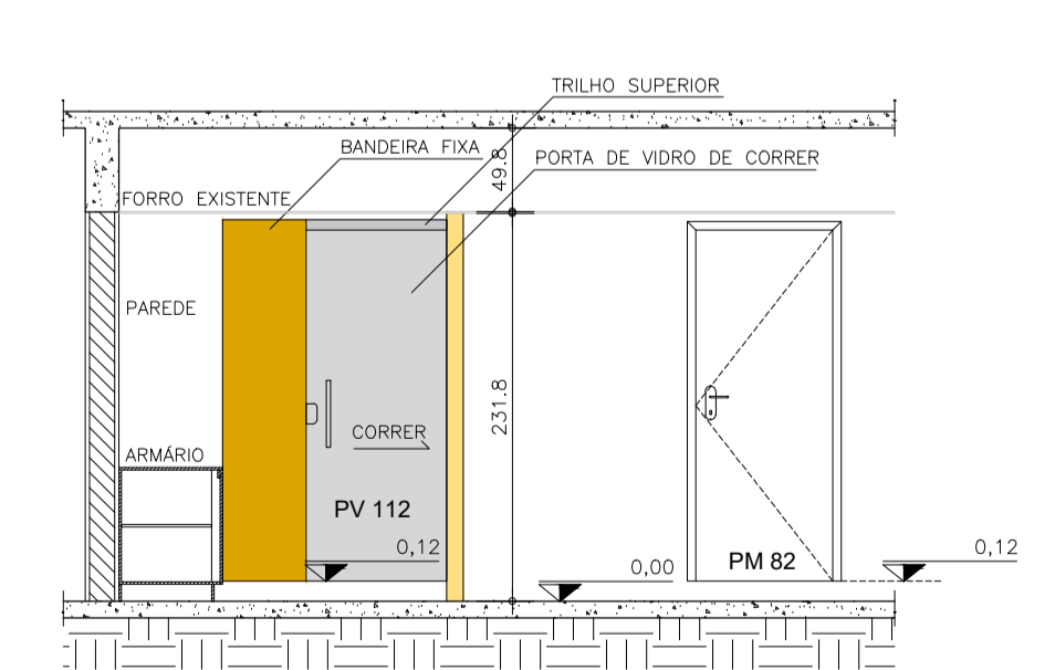
CORTE B ACESSO À SALA DO SECRETÁRIO
