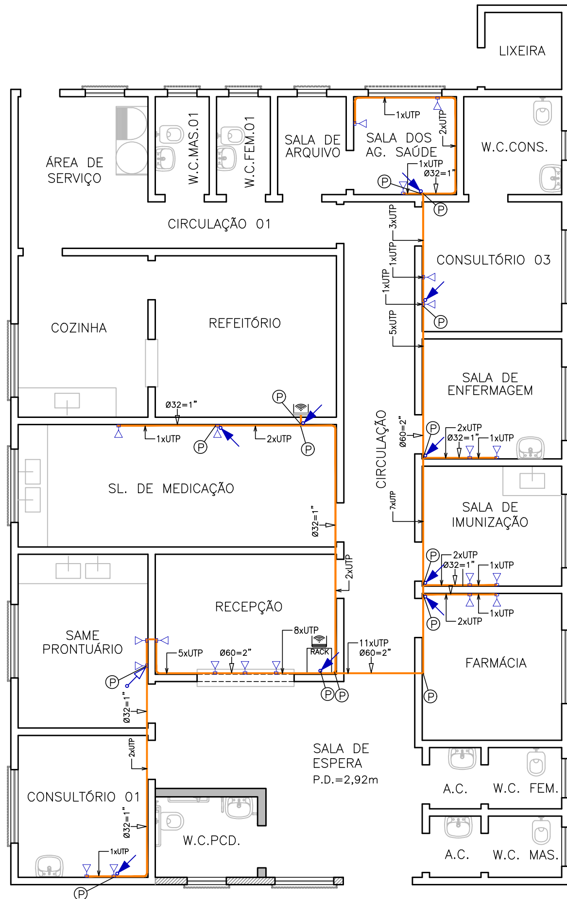
PLANTA – REDE DE LÓGICA ESC.: 1:75
